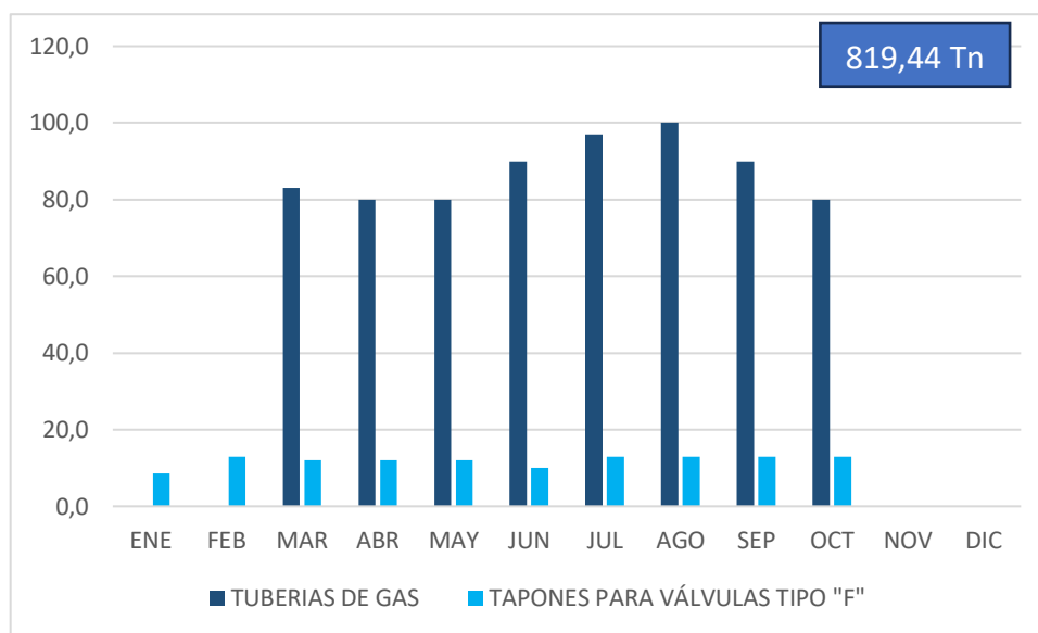
GRÁFICO 2 PROYECCIÓN DE PRODUCCIÓN DE TUBERÍAS Y TAPONES GESTIÓN 2024
